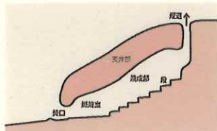
高丘古窯復元図
