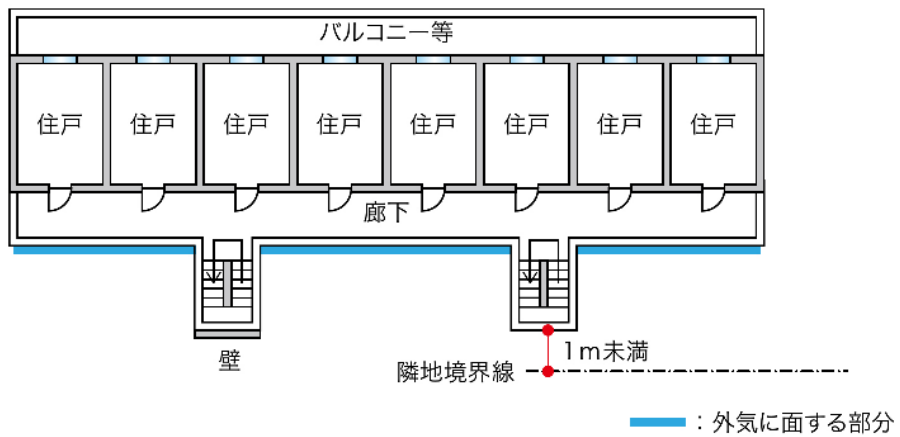
立面図
