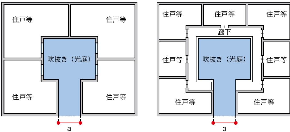
a \geq 光庭の周長のおおむね1/8、かつ、 a \geq 2m
