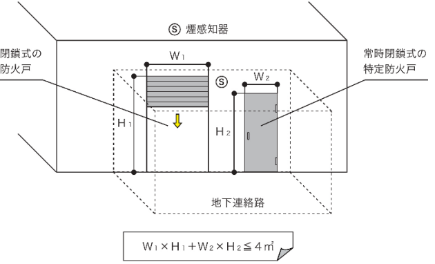
(随時閉鎖式の特定防火戸を設ける場合の例)
