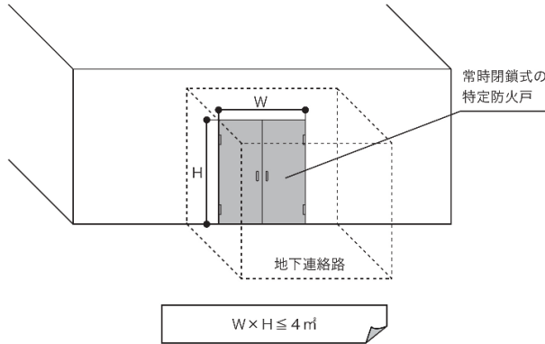
(常時閉鎖式の特定防火戸を設ける場合の例)
