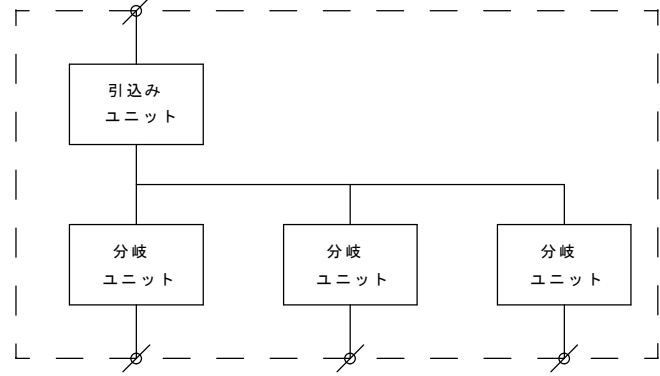
主回路構成
